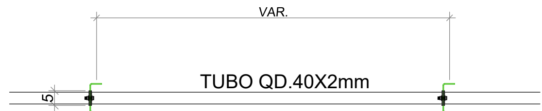
DETALHE TRAVAMENTO TERÇA/TERÇA
