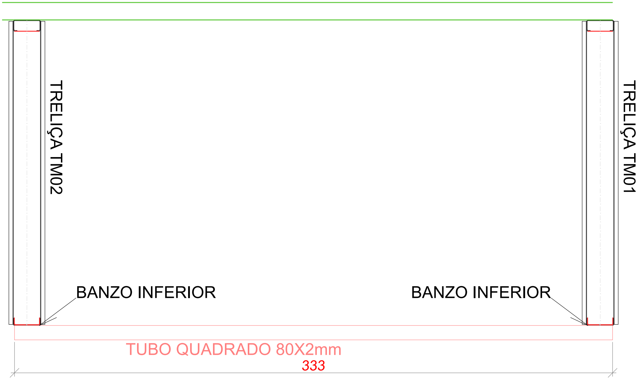
DETALHE TRAVAMENTO ENTRE TRELIÇAS 01 E 02.
